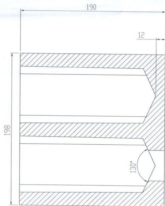
COUPE E-E ECHELLE 1 : 2
