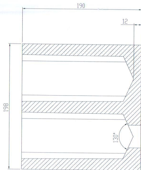
COUPE C-C ECHELLE 1 : 2
