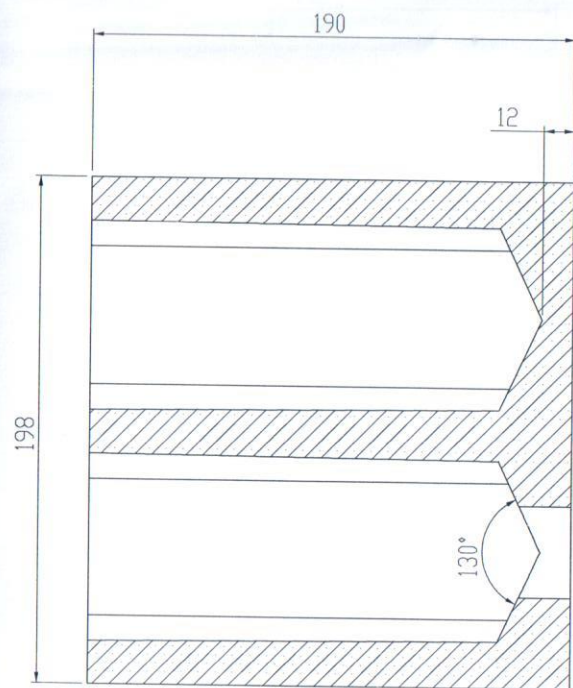
COUPE D-D ECHELLE 1 : 2
